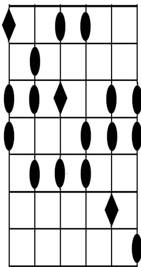
4. Dórica #4
