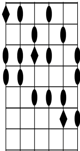
1. menor Armónica
