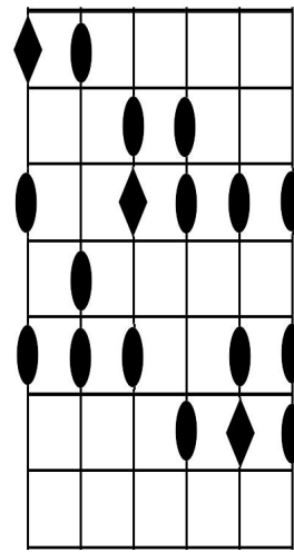
3. Jónica #5
