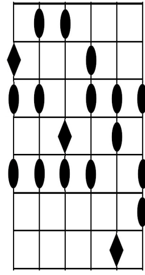
7. Armónica disminuida
